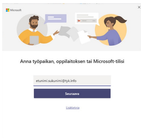
Kuva 9: Käyttäjätunnuksen syöttö
