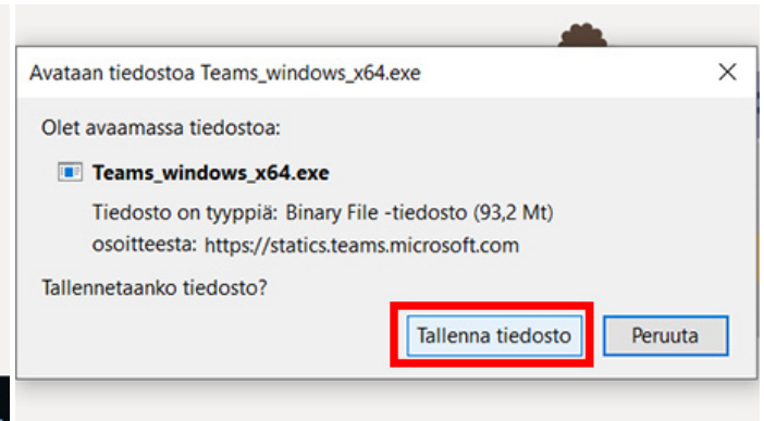
Kuva 5: Tallenna tiedosto
