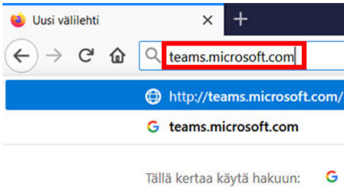
Kuva 1: Teamsin verkko-osoite
