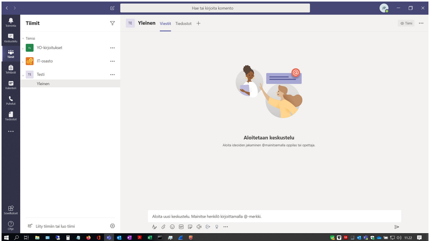
Kuva 11: Teams käyttövalmis
