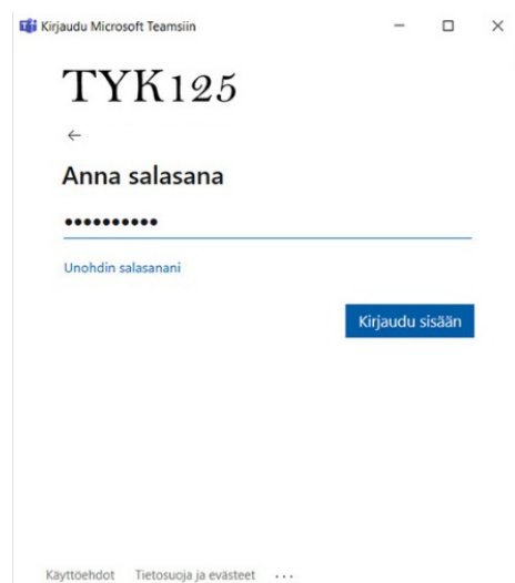
Kuva 10: Salasanan syöttö
