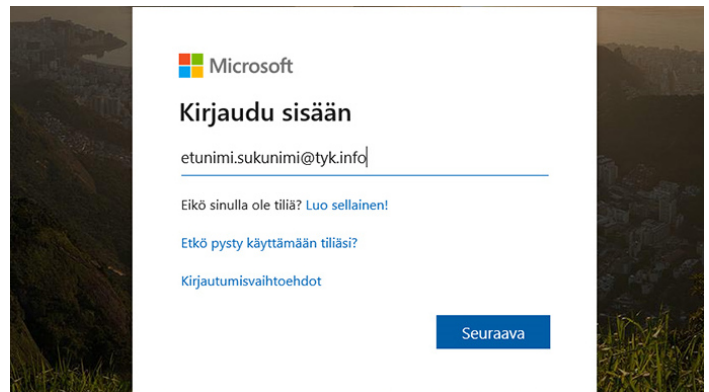
Kuva 2: Käyttäjätunnuksen syöttö
