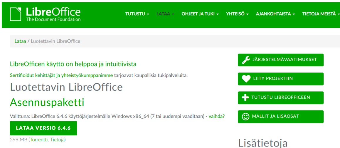
Kuva 2: Lataussivu
