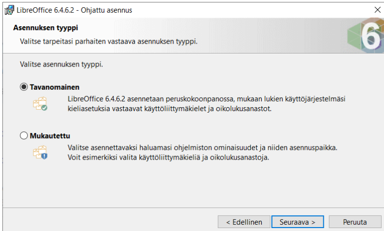
Kuva 3: Asennusvalikko
